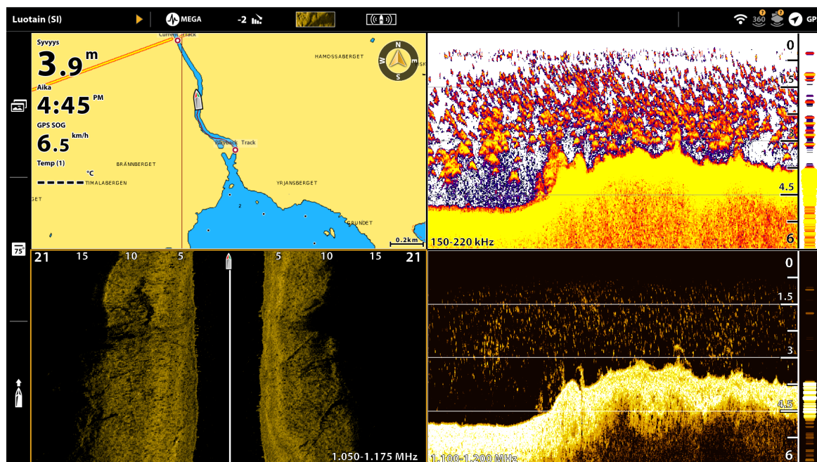
Kuva 11. Pikkalanjoessa oli lähes koko joen matkalta erittäin runsaista pikkukalamassoja, jotka erottuivat hyvin sekä 2D-kaikukuissa (oikean puolimmaisiet paneelit) että viistokaikuvassa (vasen alapaneeli).
