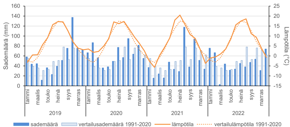
Kuva 5. Tvärminnen havaintoaseman sademäärät ja kuukauden keskilämpötilat vuosina 2019–2022 (Ilmatieteen laitos).
