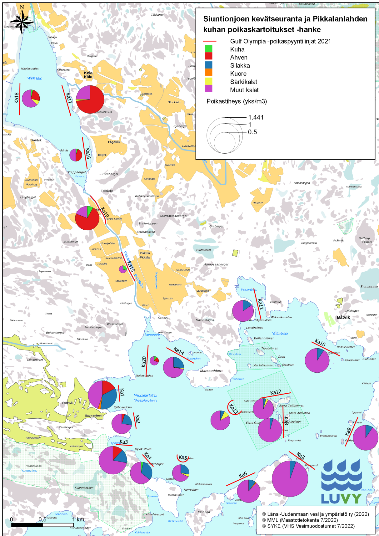
Kuva 6. Gulf-poikaspöytilinjat vuonna 2021 ja saalis lajeittain. Ympyröiden koko on suhteutettu saaliin yksilötiheyteen/m 3 .
