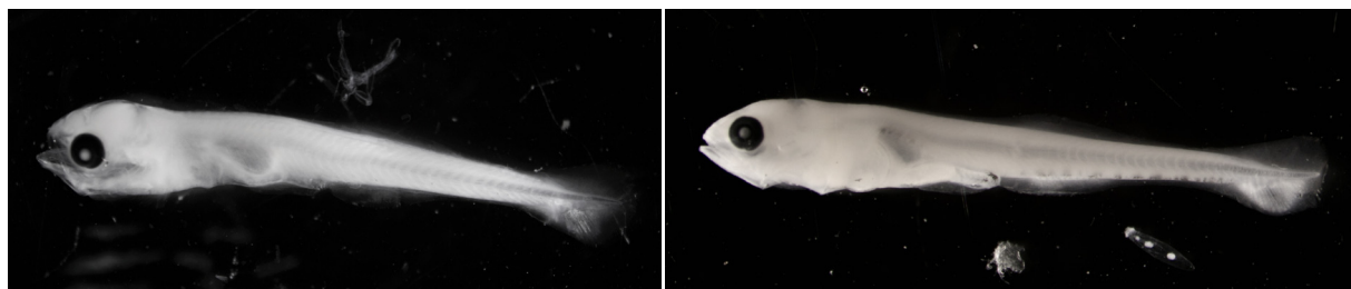
Kuva 7. Ahvenen (vasen) ja kuhan (oikea) poikanen mikroskoipituna. (LUVY / Salla Heikkinen)
