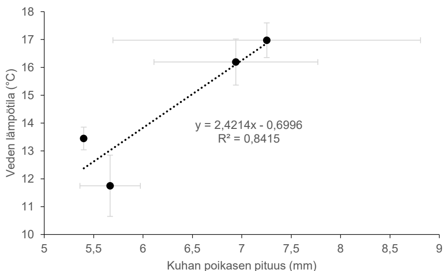
Kuva 10. Kuhan poikasen pituuden ja pohjan yläpuolisen veden lämpötilan (koko tutkimusalueen lämpötilaloggeiden keskiarvo) välinen riippuvuus. Trendi kuvaa lineaarista regressiomallia ja virhepalkit kuvaavat \pm keskihajontaa. Havaintopisteisiin on merkitty myös pyyntipäivät.
