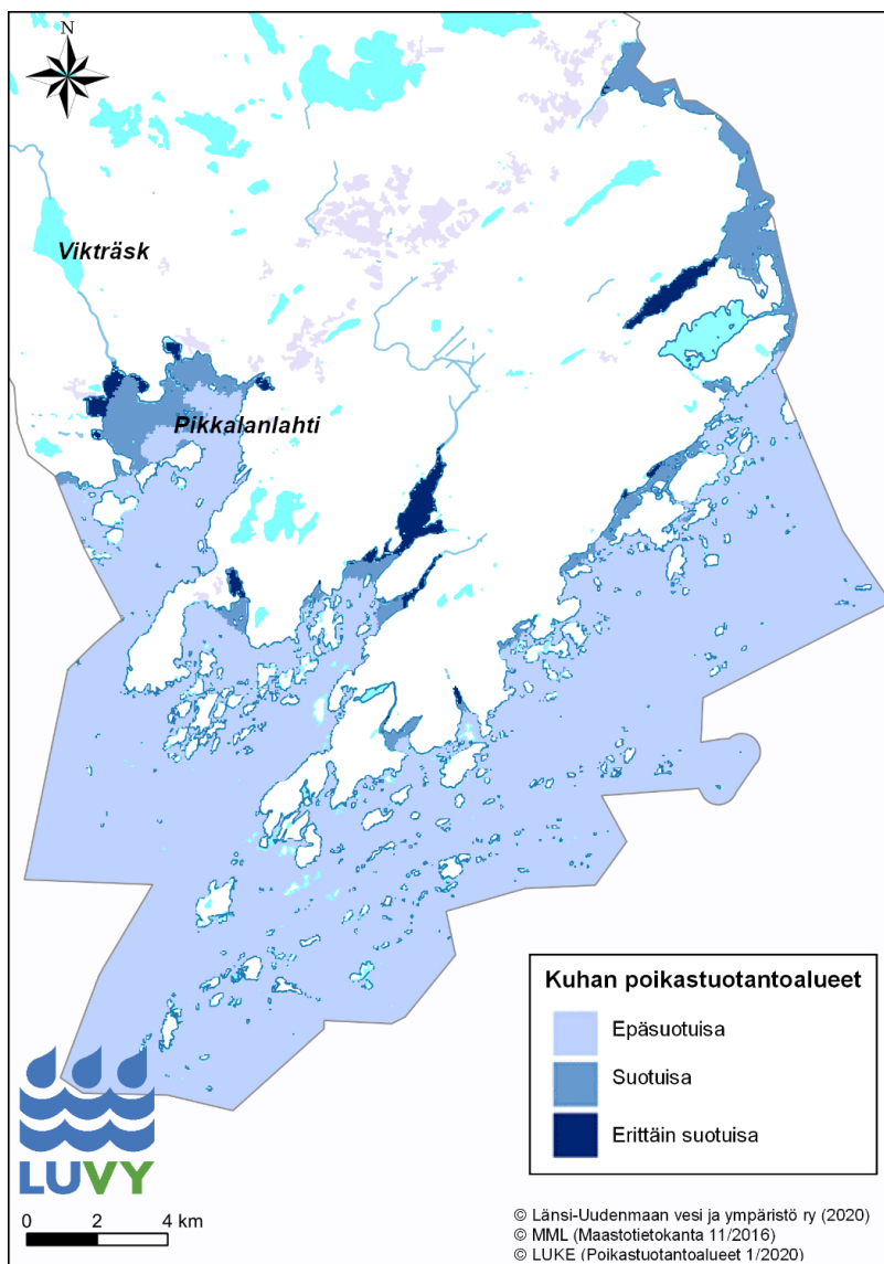
Kuva 4. Kuhan poikastuotantoalueet Kirkkonummi-Siuntionjoen kalatalousalueen merialueella VELMU-mallinnuksen perusteella. Poikastuotantoalueet on mallinnettu Luonnonvarakeskuksen toimesta vuosina 2007–2014 kerättyjen kalanpoikashavaintojen ja paikkatietomuodossa olevien ennustemuuttujien perusteella. Menetelmä on kuvattu tiedejulkaisussa Kallasvuo ym. (2016).
